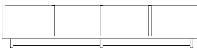
Plank Bookcase Low H: 50,5 x W: 40 x L: 220 cm
